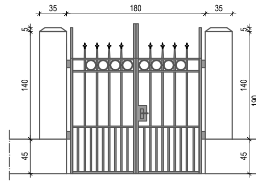
КАПИЈА ЗА ЂАКЕ СА СТУБОВИМА новопројектовано решење
