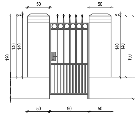
ДЕТАЉ ГЛАВНЕ КАПИЈЕ новопројектовано решење
