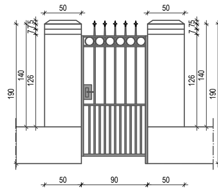
ДЕТАЉ ГЛАВНЕ КАПИЈЕ СА СТУБОВИМА постојеће стање
